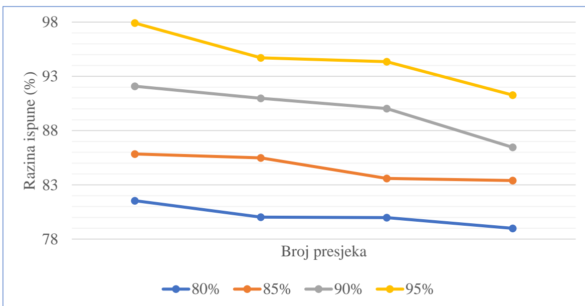
Slika 72. Razina ispune za presjeke modela sa 8 spona
