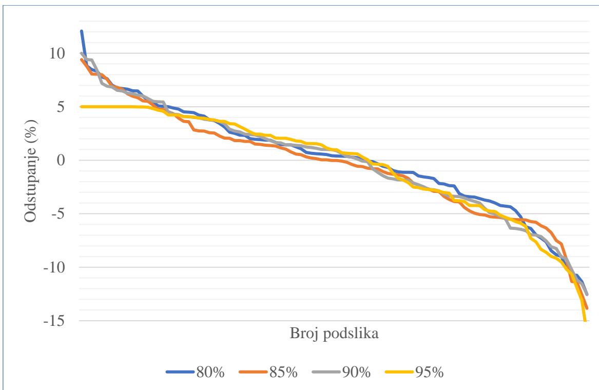
Slika 71. Odstupanje razine ispune podslika za modele sa 8 spona
