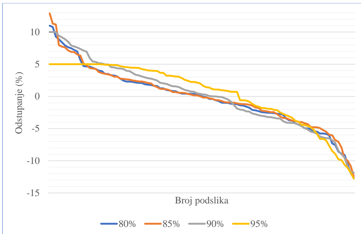
Slika 83. Odstupanje razine ispune podslika za modele sa 10 spona
