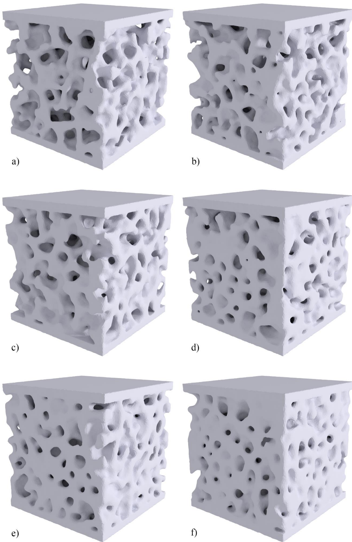
Slika 151. Poligonalni modeli sa razinom ispune od 50 do 75%
