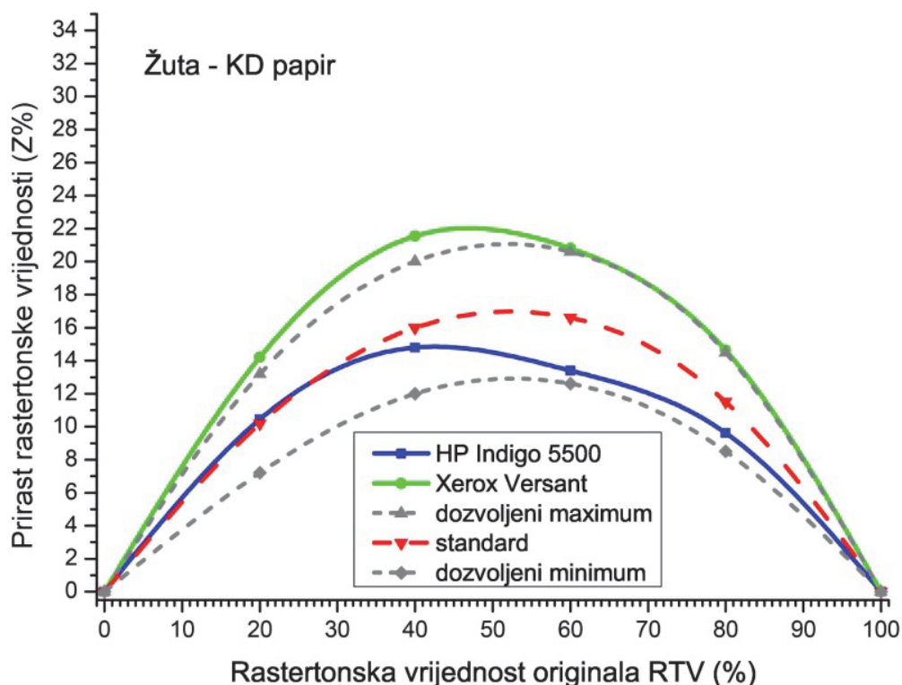
Slika 18 - Krivulja reprodukcije žutih otisaka na papiru za umjetnički tisak
