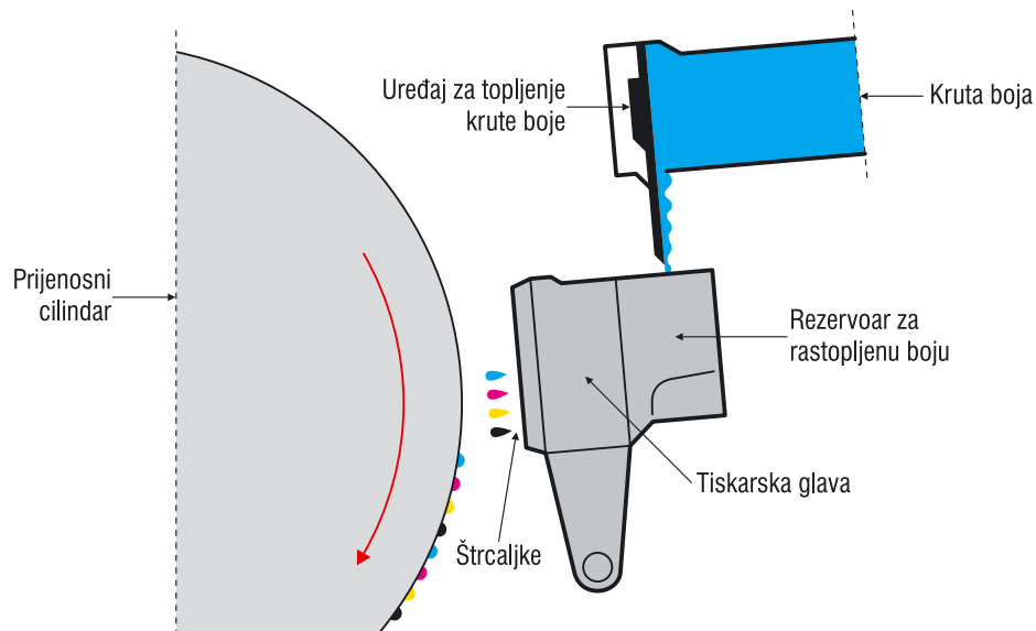
Slika 4. Transformacija boje i njezino nanošenje na prijenosni cilindar kod hot melt inkjet tehnologije
