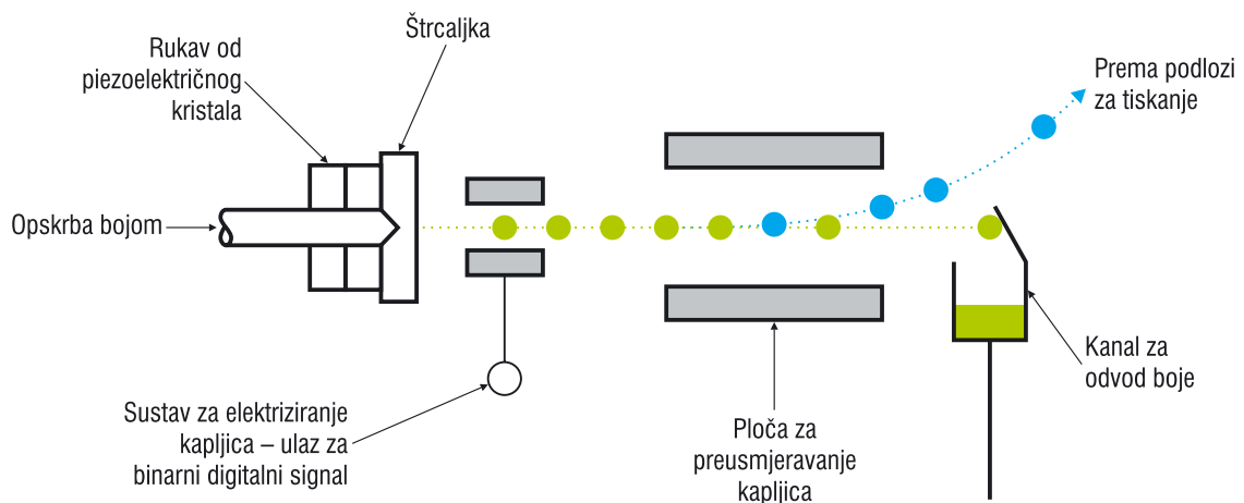
Slika 1. Binarni kontinuirani piezzo inkjet
