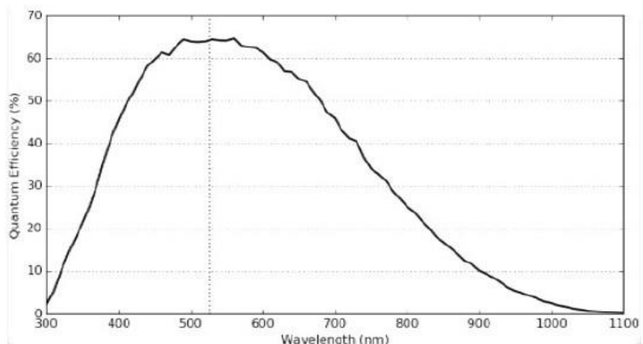
Slika 13: Prikaz osjetljivosti senzora multispektralne kamere (monokromatska) (izvor: Multispektralna slikovna analiza pisane kulturne baštine dr.sc. Vladimir Cviljušac , prof. dr. sc. Damir Modrić, dr.sc. Alan Divjak 6.9.2022. Hrvatski državni arhiv)
