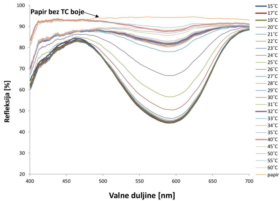
Slika 21. Krivulje spektralne refleksije pri izlaganju TK otiska na sintetičkom papiru postepenom povećanju temperature ( )
