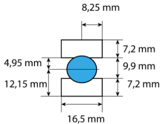
Slika 12. Presjek ležaja
