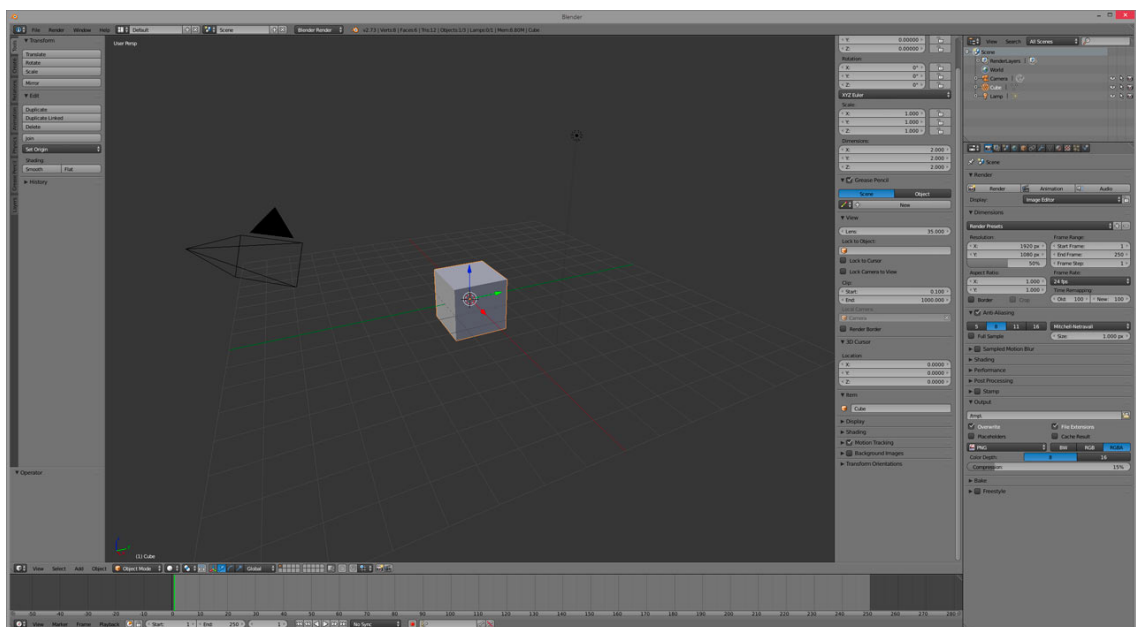
Slika 5. Sučelje Blendera
