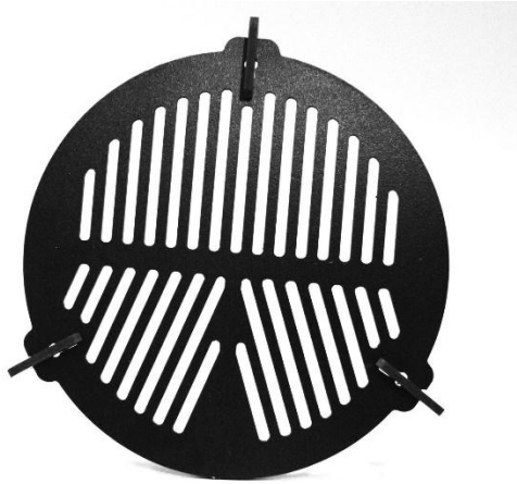
Slika 10 Bahtinova maska
