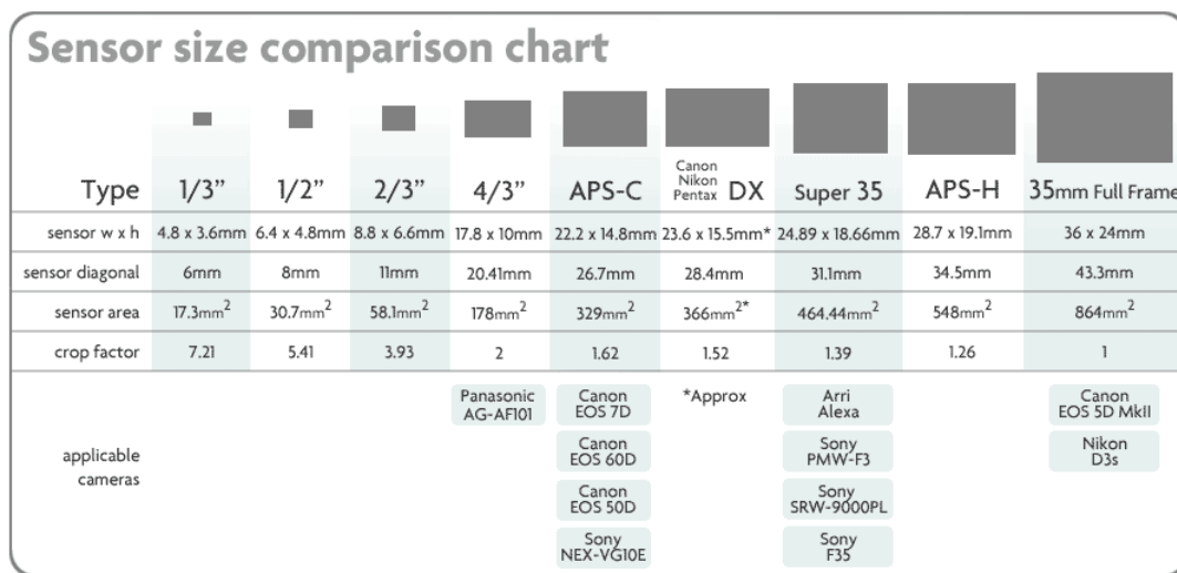
Slika 6. Veličina senzora
