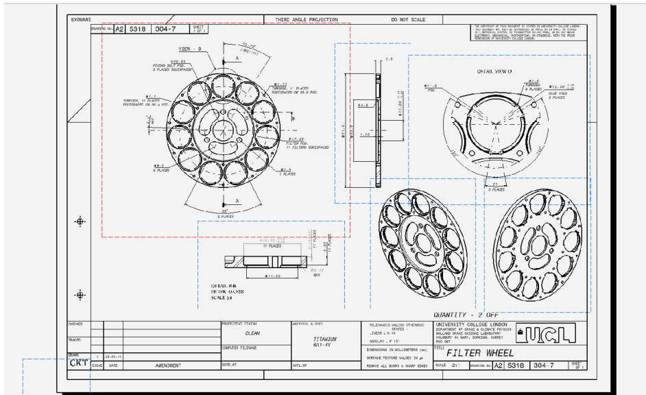
Slika 13. - CAD crtež [12]
