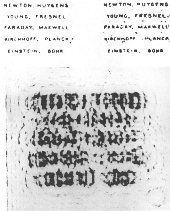
Slika 2. Jedan od Gaborovih prvih holograma [4]
