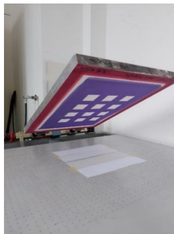
Slika 15 - Sitotiskarski stroj za ručno otiskivanje (Autorska slika)
