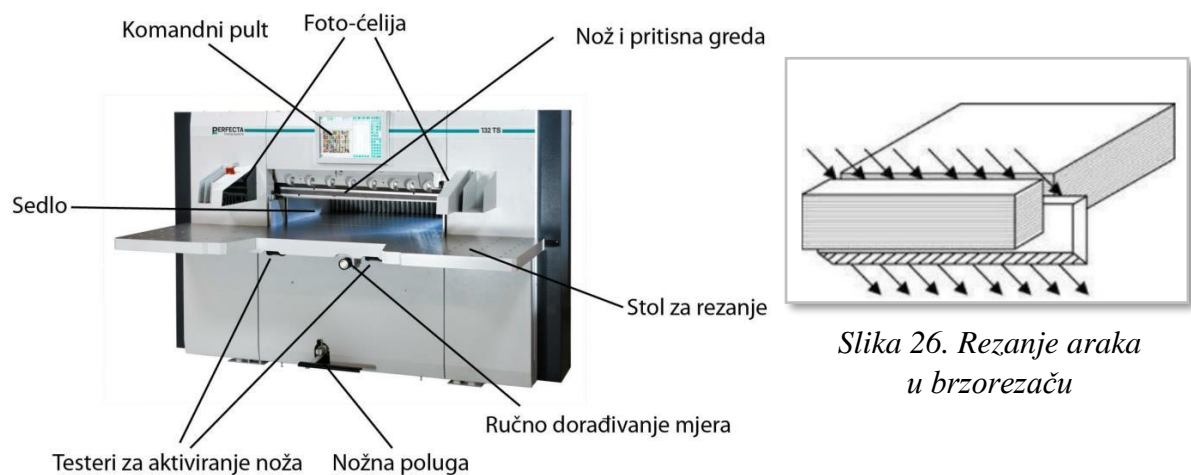
Slika 25. Brzorezač
