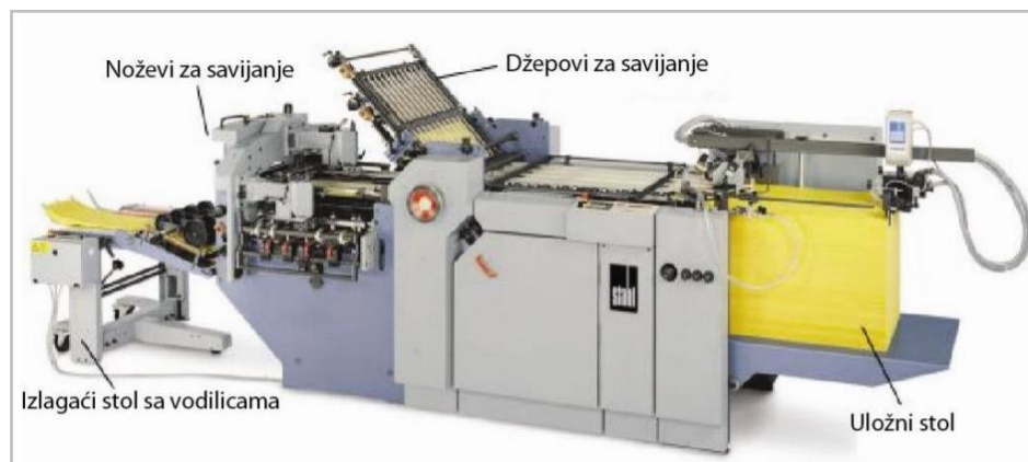
Slika 31. Karakteristike savijačice
