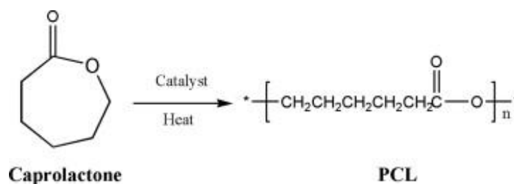
Slika 15. Polikaprolakton
