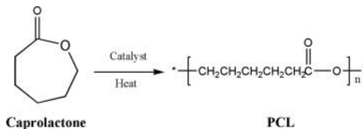
Slika 15. Polikaprolakton
