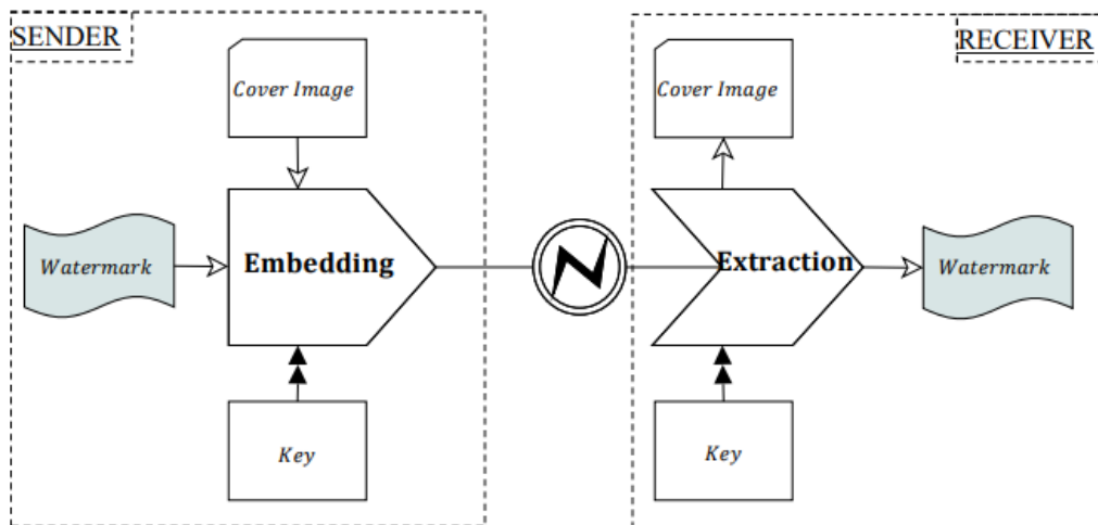
Slika 4. Shema distribuiranja digitalnog vodenog žiga
