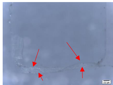
Slika 6.10 Mikroskopska snimka POM-a, mehaničko graviranje, rubni dio kvadratnog oblika
