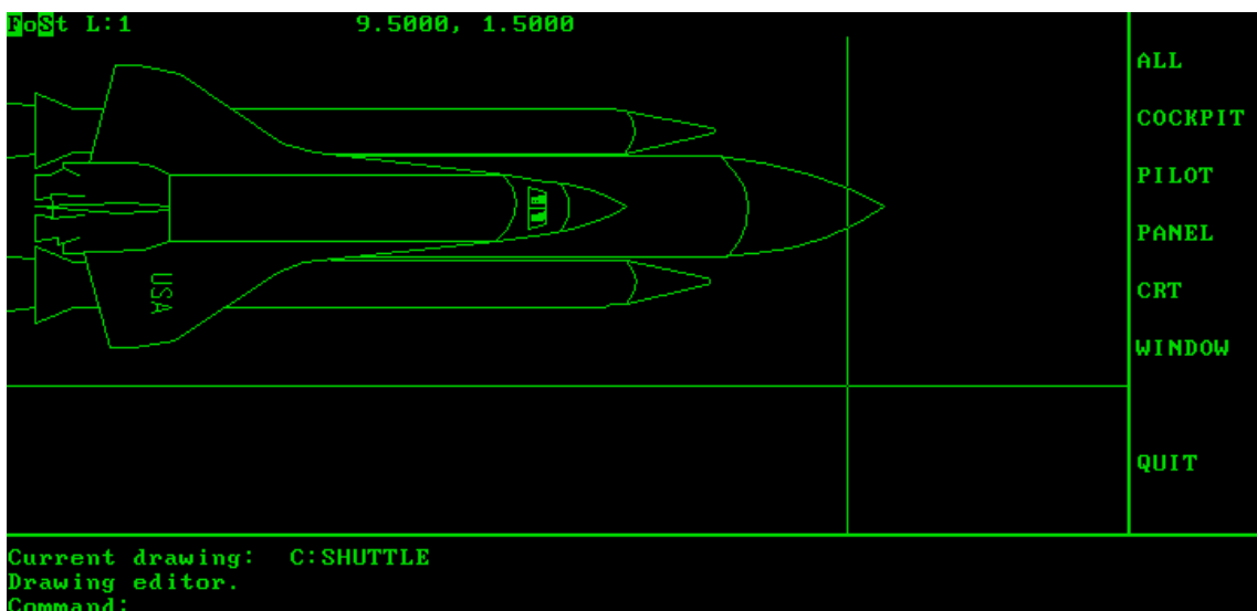
Slika 4. AutoCAD Version 1.0
