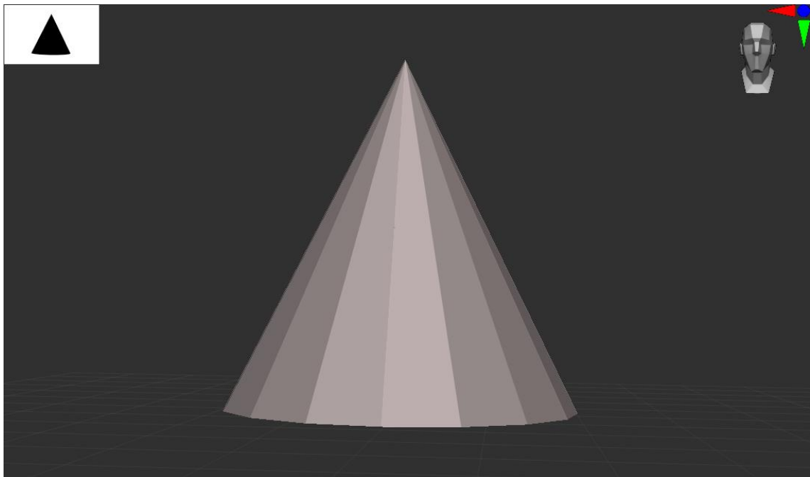
Slika 34. Stožac
