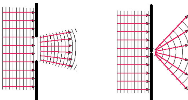
Slika 56: Difrakcija
