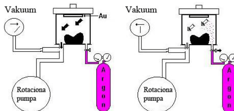
Slika 34. Uređaj za napanivanje [60]
