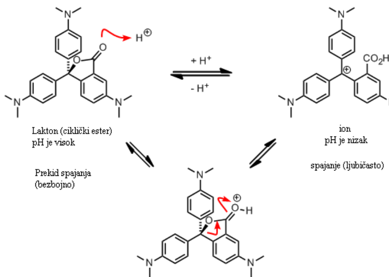
Slika 21. Spajanje aromatskih prstenova [43]
