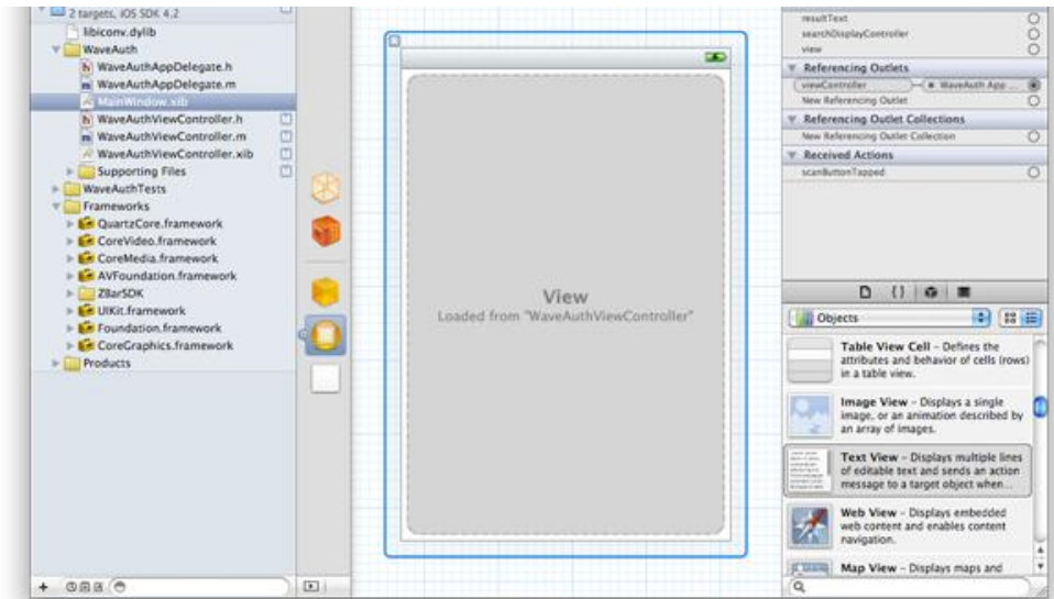
Slika 2.4 Xcode 4 sučelje
