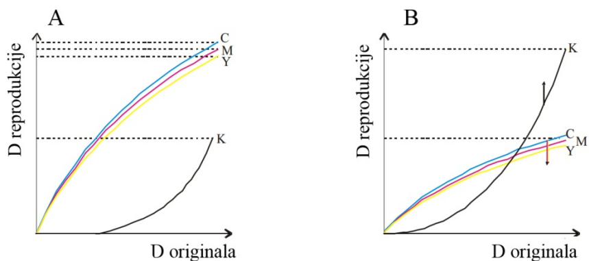
Slika 13. Nanosi bojila: A) bez UCR metode, B) s UCR metodom
