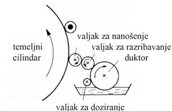
Slika 3. Osnovni princip uređaja za vlaženje kod ofsetnih strojeva [3]
