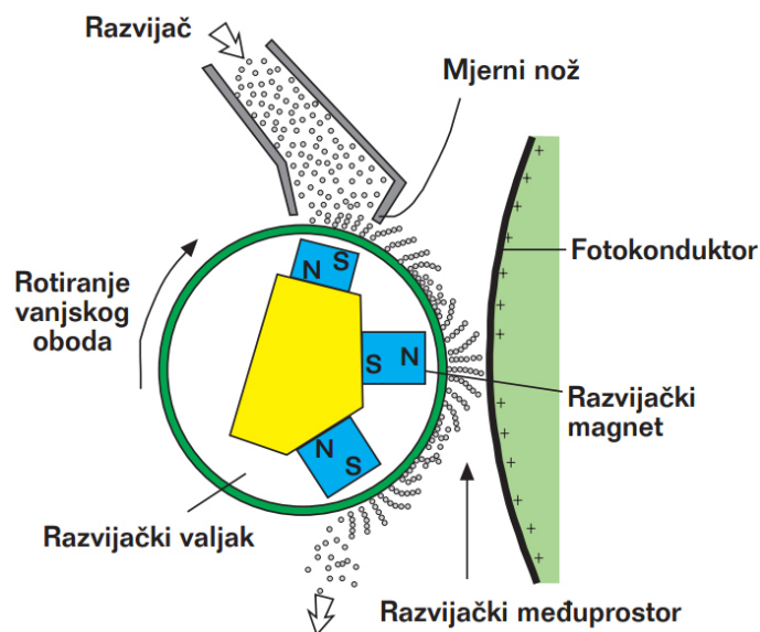
Slika 10. Razvijanje dvokomponentnog tonera magnetskom četkom (Izvor: I. Majnarić, Studija indirektno elektrofotografije, doktorska disertacija, 2007.)
