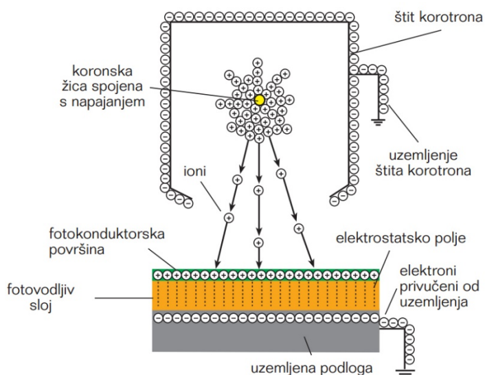
Slika 5. Shematski prikaz principa pozitivskog nabijanja (korotronom) (Izvor: I. Majnarić, Studija indirektno elektrofotografije, doktorska disertacija, 2007.)
