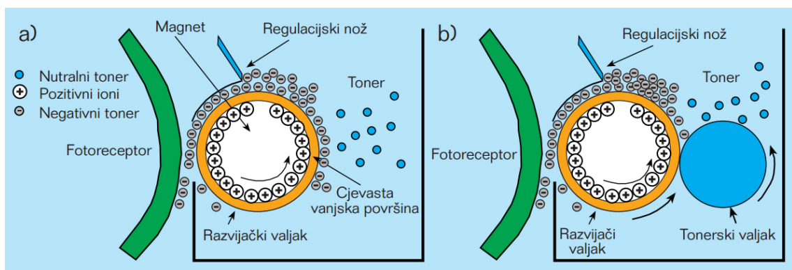
Slika 9. Razvijanje jednokomponentnog tonera: a) razvijačka jedinica sa razvijačkim valjkom s permanentnim magnetom, b) razvijačka jedinica sa razvijačkim valjkom i tonerski valjak (Izvor: I. Majnarić, Studija indirektno elektrofotografije, doktorska disertacija, 2007.)
