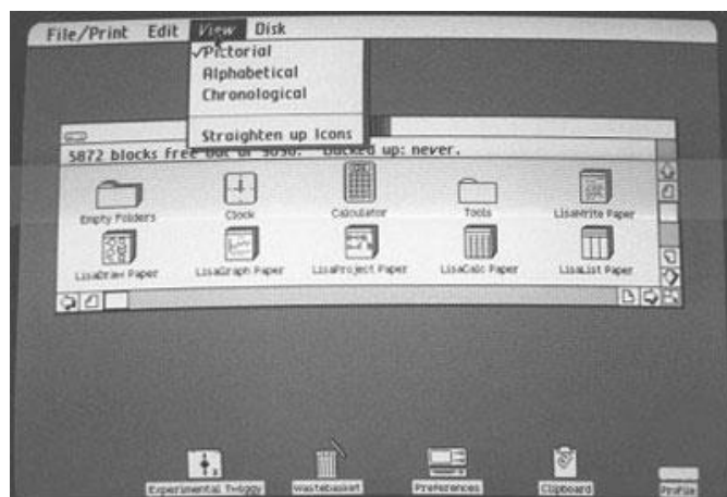
Slika 3. Grafičko korisničko sučelje Lisa računala ( http://origin.arstechnica.com/images/gui/10-Lisa1.jpg )
