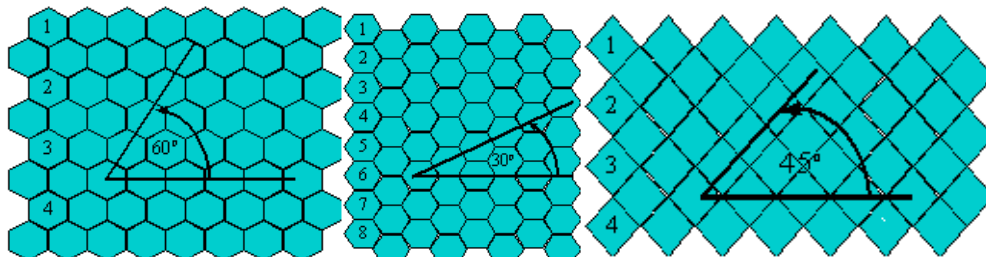
Slika 12. Kutevi ćelija aniloks valjka
