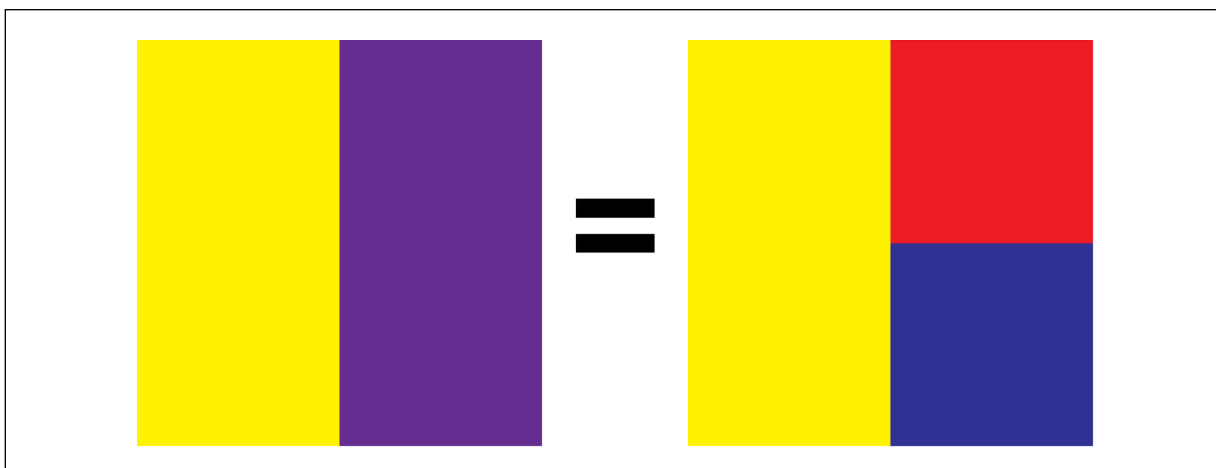
Slika 24: Trozvuk primara
