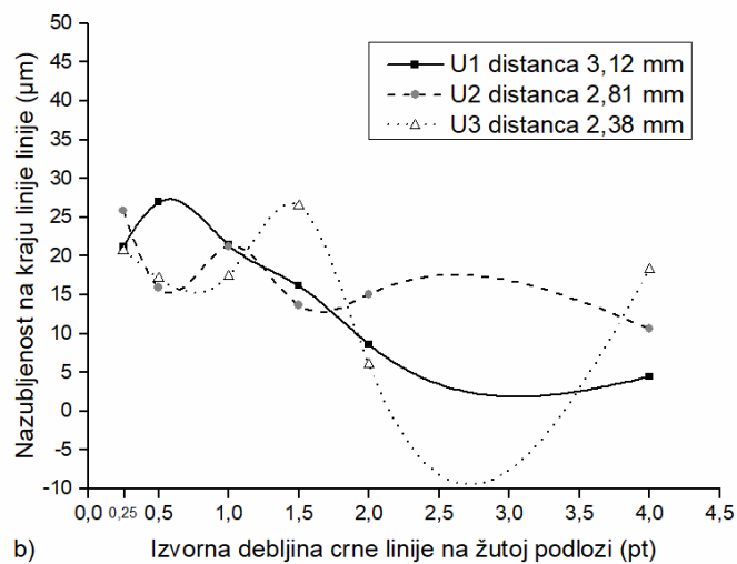
Slika 46. Krivulje zamrljanosti nastale eksperimentalnim pomicanjem ispisne glave Inkjet printera a) na početku crne linije na kontrastnoj žutoj podlozi, b) na kraju crne linije na kontrastnoj žutoj podlozi
