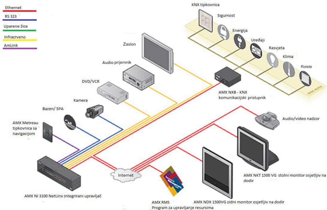
Slika 4. Konnex protokol
