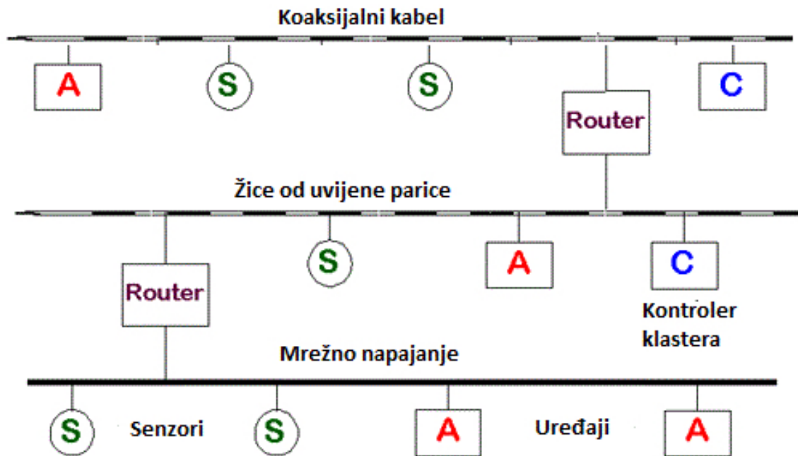
Slika 3. CEBus protokol
