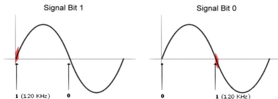
Slika 1. X-10 protokol
