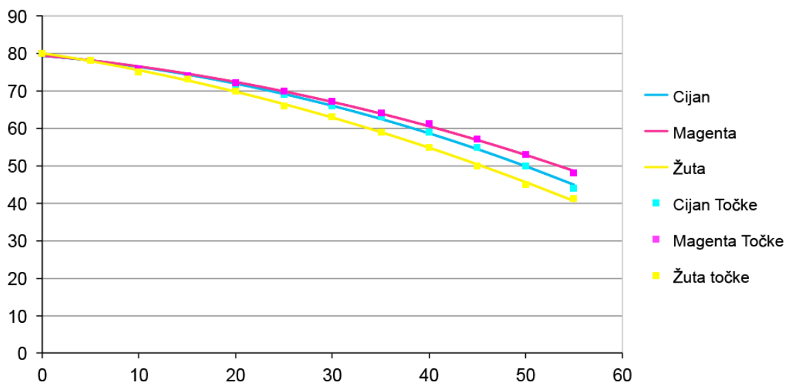
Grafikon 2. Prikaz pada vrijednosti Cijana, Magente i Žute u odnosu na povećanje Crne boje prema vrijednostima u Tablici 2.
