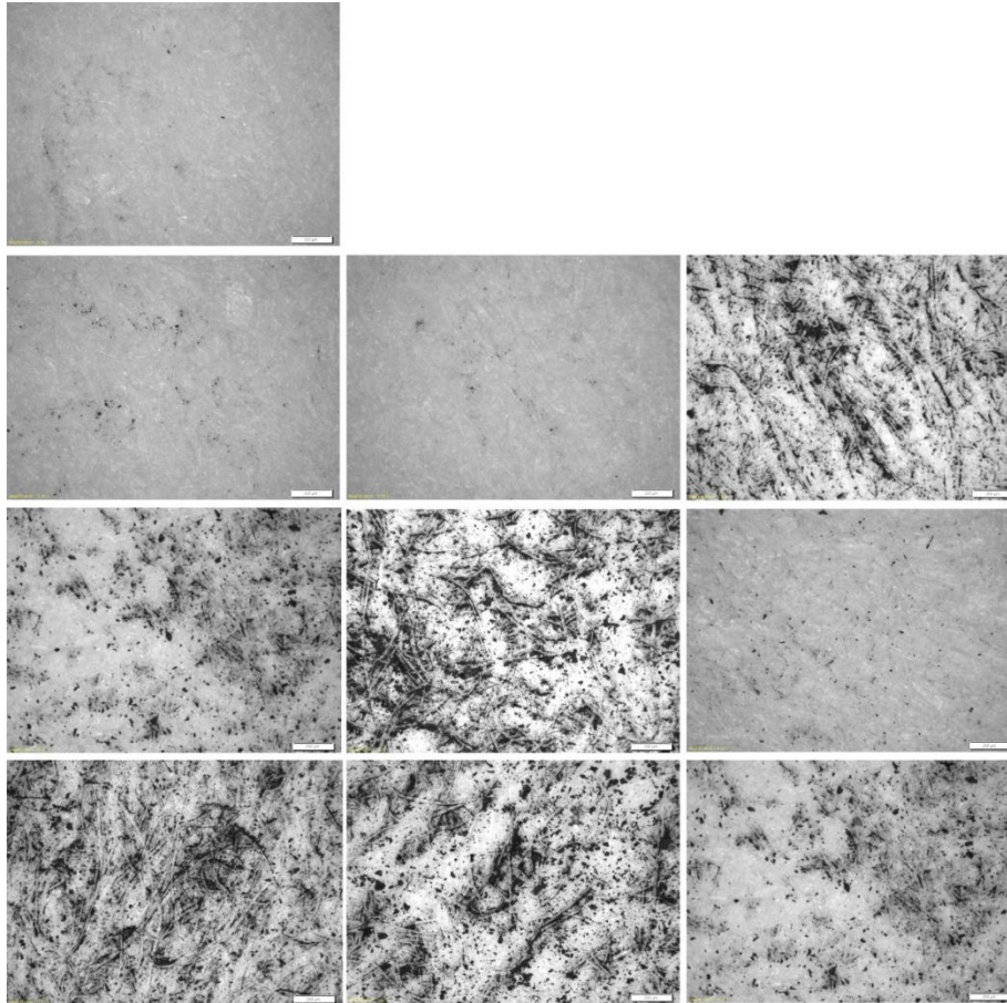
Slika 30. Mikroskopski prikaz otiranih površina na ofsetnom papiru za premazani papir: a) boja bez dodatka nanočestica, b) 0, 1 i 1,5% TiO 2 (anatas), c) 0, 1 i 1,5% TiO 2 (rutil), d) 0, 1 i 1,5% ZnO
