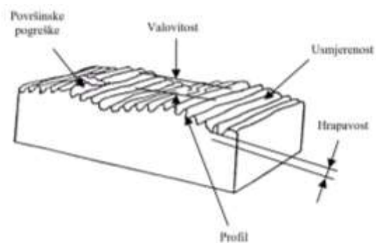
Slika 44 Odstupanja površine
