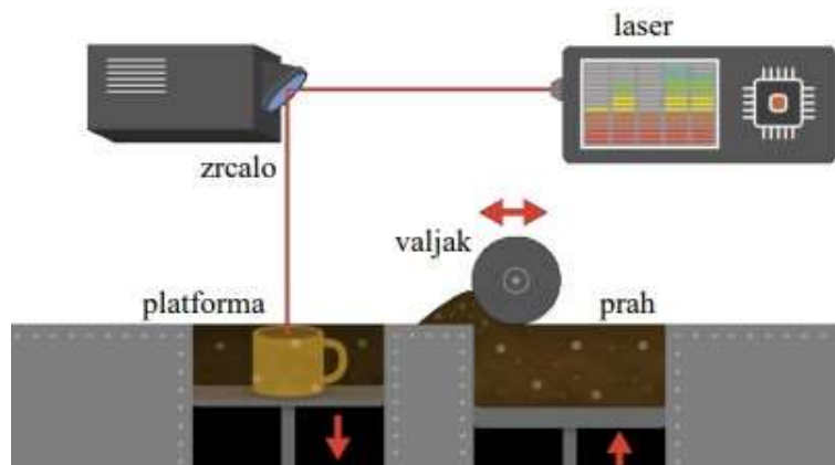
Slika 24 Selektivno lasersko srašćivanje [15]
