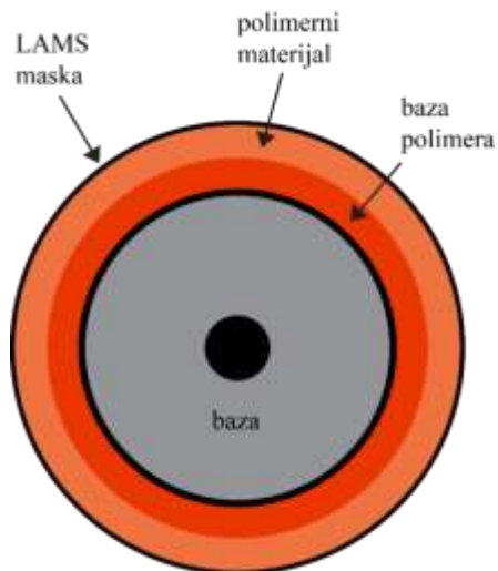
Slika 15 Presjek ovojne tiskovne forme s LAMS maskom
