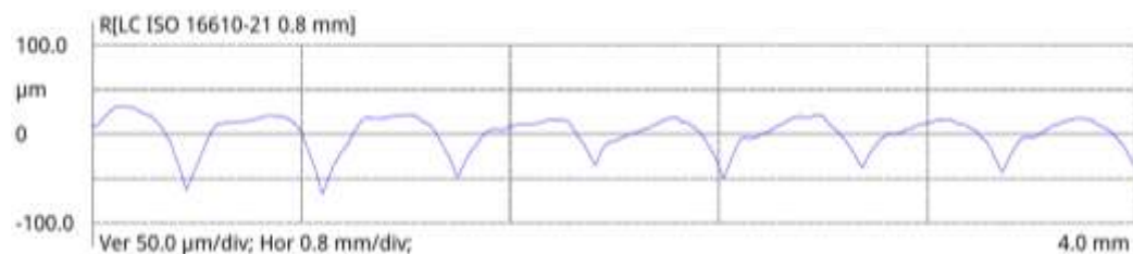
g) PLA/PCL/SiO 2 50/50/1%
