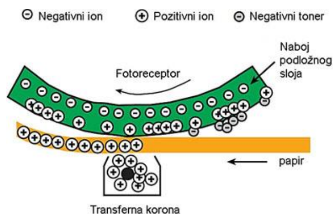
Slika 12. Transfer tonera - djelovanje transferne korone [Izvor: I. Majnarić, Studija indirektno elektrofotografije, doktorska disertacija, 2007.]
