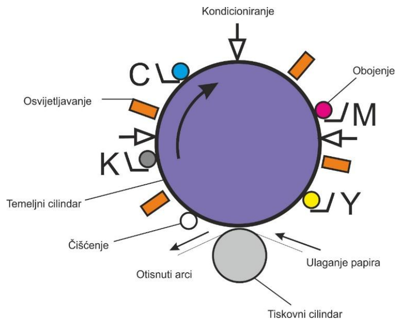
Slika 4. Satelitski direktni, jednoprolazni, višebojni sistem (I. Majnarić, Studija indirektna elektrografije, doktorska disertacija, 2007., str 56.)
