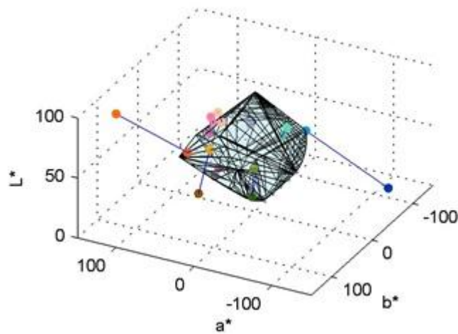
Slika 21: Mapiranje gamuta
