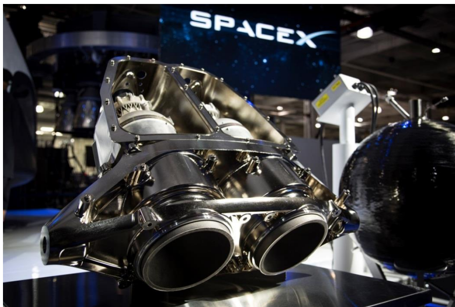
Slika 24. SuperDraco raketni motor izrađen 3D aditivnom tehnologijom
