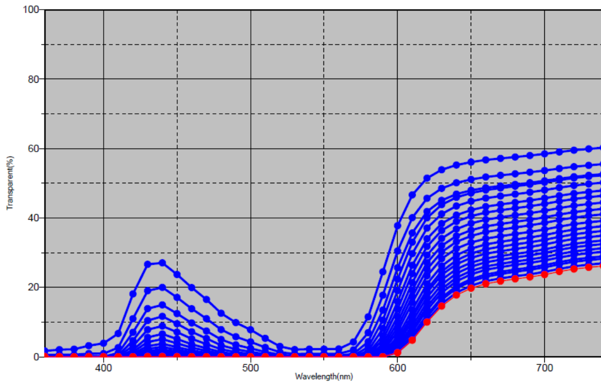
Slika 64 Spektralne krivulje transmissijskih svojstava ispitnih uzoraka s magenta bojilom
