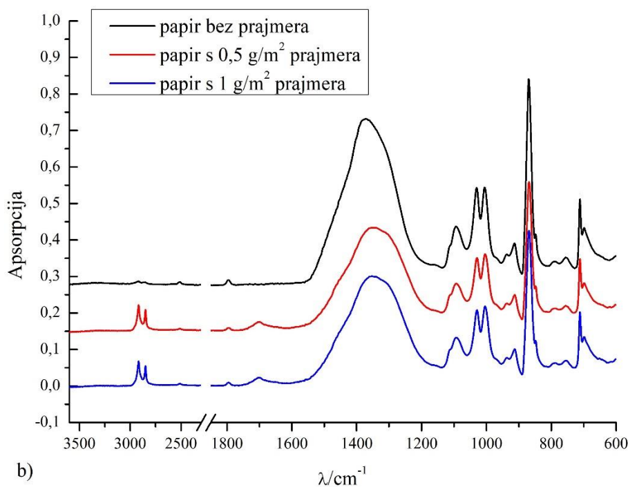
Slika 49. Prikaz FTIR-ova izmjerenih uređajem „Shimadzu IRAffinity-1” na papiru za umjetnički tisak Condac: a) prije oplemenjivanja, b) nakon oplemenjivanja prajmerom (0,5 g/m 2 i 1 g/m 2 )
