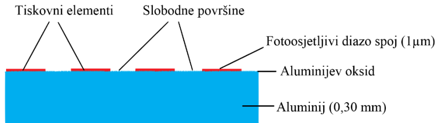
Slika 38. Presjek tiskovne forme za ofsetni tisak
