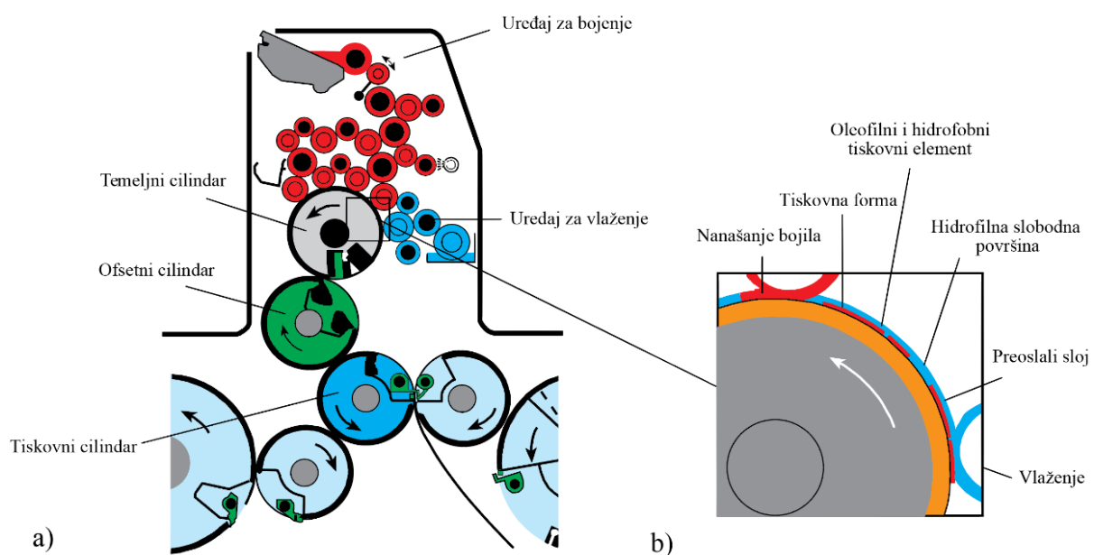
Slika 39. Tiskovna jedinica za ofsetni tisak: a) konstrukcija s tri cilindra, b) zona nanašanja tekućine za vlaženje i bojila
