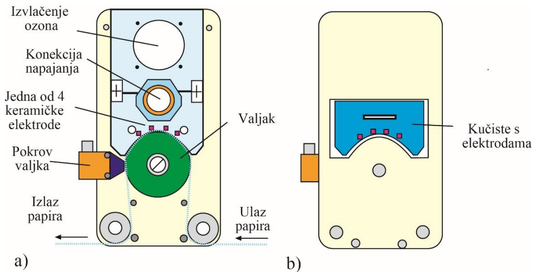
Slika 14. Vetaphone korone upotrijebljene u HP Indigo stroju: a) stražnja strana, b) prednja strana
