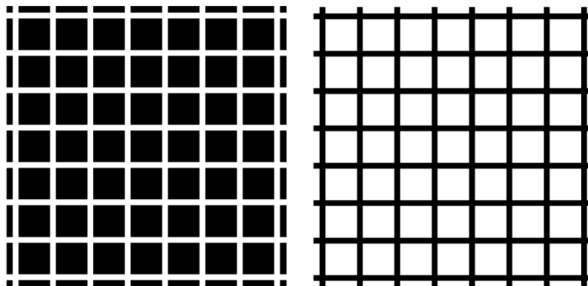
Slika 2.44. Hermannov efekt
