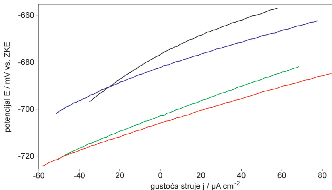
Slika 55. Krivulje linearne polarizacije čelika u elektrolitima: 8 EKO (—), 9 EKO-TV(—), 19 EKO-OFF/RO (—) i 16 EKO-TV-OFF/RO (—)
