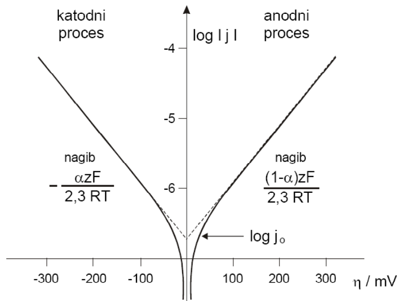
Slika 6. Struja-potencijal karakteristike za elektrokemijsku reakciju pod aktivacijskom kontrolom
