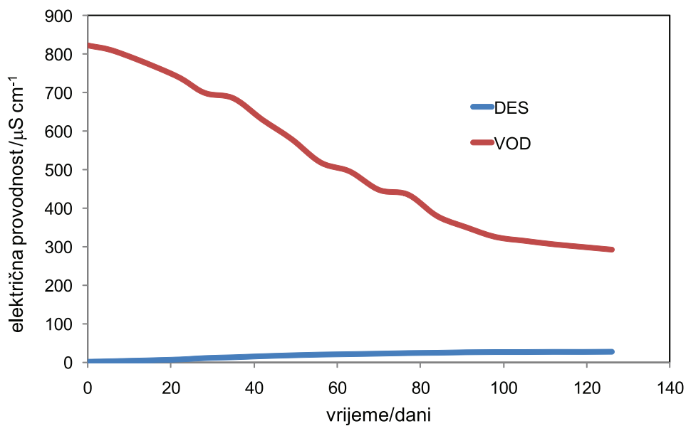
Slika 20. Promjena električne provodnosti destilirane i vodovodne vode s uronjenim čeličnim uzorkom kroz vremensko razdoblje od 126 dana
