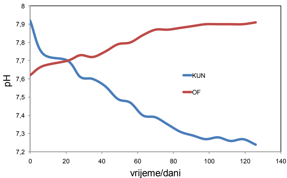
Slika 19. Promjena pH vrijednosti vodene otopine spojeva s površine glatko premazanog papira KUN i vodene otopine spojeva s površine nepremazanog papira OF s uronjenim čeličnim uzorkom kroz vremensko razdoblje od 126 dana
