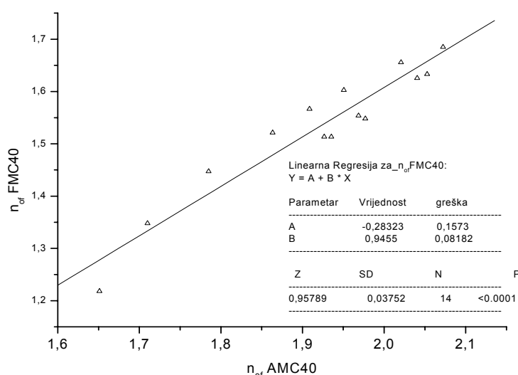
Slika 76 Korelacija vrijednosti parametra n za cijan tiskan amplitudno i frekventno moduliranim rasterom na ofsetnoj tiskovnoj podlozi za F=40\% od 570 do 700nm.
