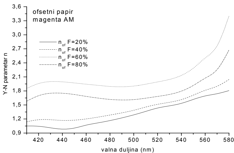
Slika 64b Parametar n kao funkcija valne duljine i rastertonske pokrivenosti bojilom, za ofsetnu tiskovnu podlogu otisnutu magentom, amplitudno moduliranim rasterom od 80lin/cm.
