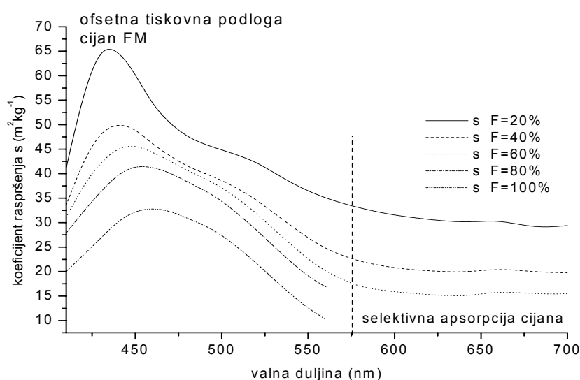
Slika 70a Koeficijent raspršenja kao funkcija valne duljine i rastertonske vrijednosti za cijan. U području selektivne apsorpcije cijana za F=80 i 100\% vrijednosti koeficijenta raspršenja nisu realne.
