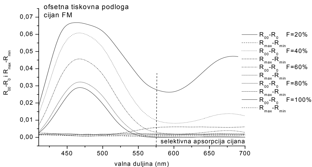
Slika 68a Razlika mjerenih refleksijskih spektara na snopu od 20 uzoraka, R_\infty i na crnoj podlozi, R_0 , R_\infty - R_0 , te područje rasipanja mjerenih veličina za cijan R_{\text{Range}} = R_{\max} - R_{\min} kao funkcija valne duljine i rastertonske vrijednosti ( F=20-100\% ).
