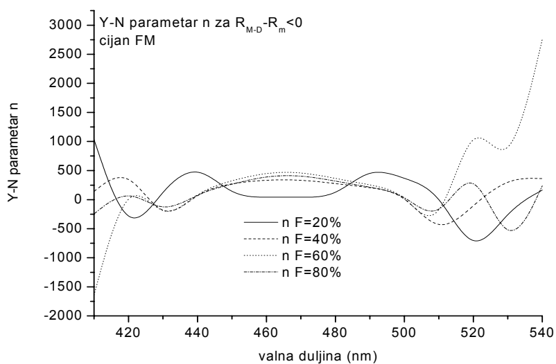
Slika 62b Rješenja transcendentne jednadžbe za parametar n rastertonskih vrijednosti F=20, 40, 60 i 80\% u području dominantne refleksije cijana za \Delta R < 0 .
