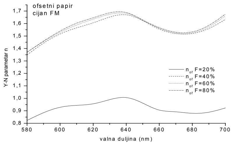
Slika 63a Yule-Nielsenov parametar n kao funkcija rastertonske vrijednosti i valne duljine u području selektivne apsorpcije cijana.
