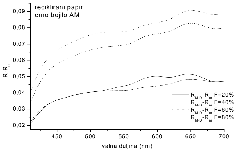
Slika 57b Razlika računskih i mjenih refleksijskih spektara ( \Delta R = R_{M-D} - R_m ) za crno bojilo kao funkcija valne duljine i rastertonske vrijednosti.
