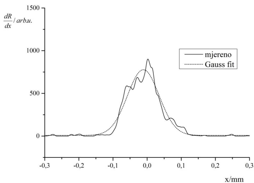
Slika 149. Epson Stylus Photo 2400 - profil optičkog prirasta rastertonske vrijednosti za liniju nominalne debljine 1 mm otisnute na a) uredskom papiru b) ofsetnom papiru c) papiru za digitalni tisak
