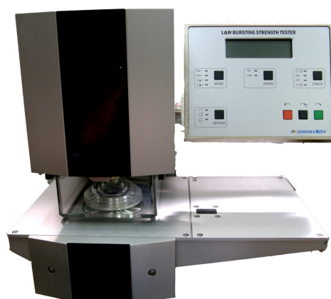
Slika 16. Mullen tester proizvođača Lorentzen & Wettre
