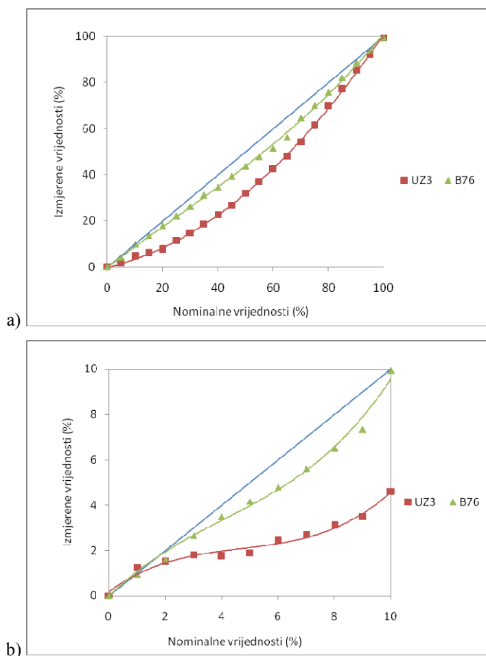
Slika 70. Pokrivenost površine nominalnih i izmjerenih vrijednosti za uzorke tiskovnih formi s bump-up krivuljom i krivuljom prilagođenom za proizvod 3 (Uzorak 3) kod linijature 76 \text{lin cm}^{-1} a) od 0 do 100%; b) od 0 do 10% pokrivenosti površine
