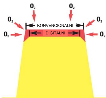
Slika 18. Prikaz razlike u obliku tiskovnih elemenata dobivenih konvencionalnim i digitalnim postupkom
