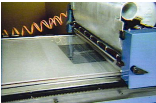
Slika 9. Izrada fotopolimerne tiskovne forme
