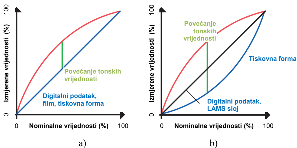
Slika 44. Krivulje reprodukcije tonova a) konvencionalne tiskovne forme i b) CtP tiskovne forme
