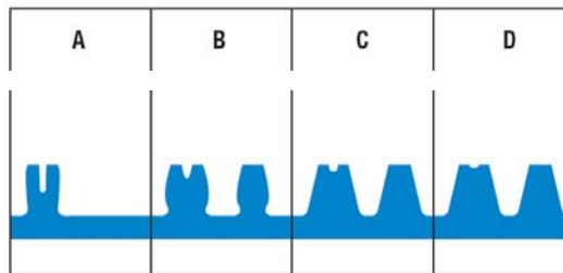
Slika 40. Prikaz bočnog dijela tiskovnog elementa i srednje dubine reljefa u ovisnosti o trajanju glavne ekspozicije
