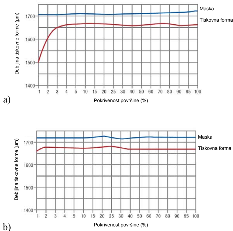
Slika 46. Prikaz promjene u debljini tiskovne forme u ovisnosti o pokrivenosti površine
