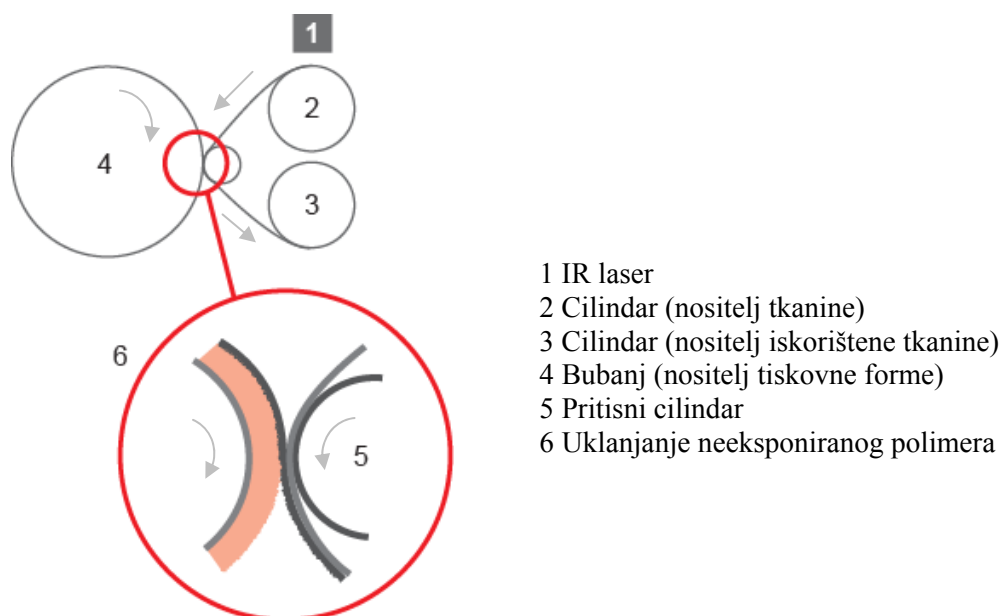
Slika 17. Termalna jedinica
