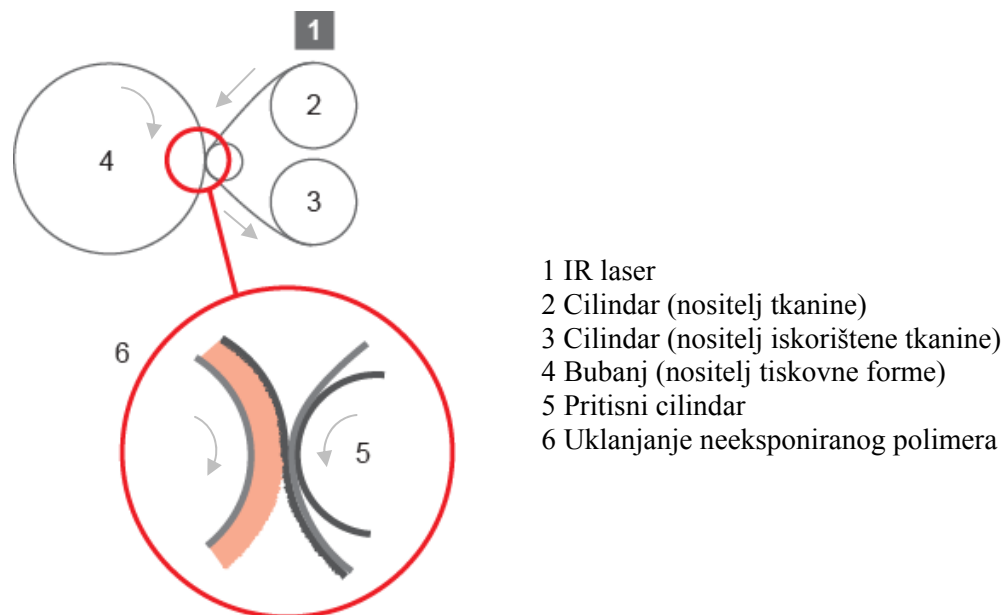
Slika 17. Termalna jedinica
