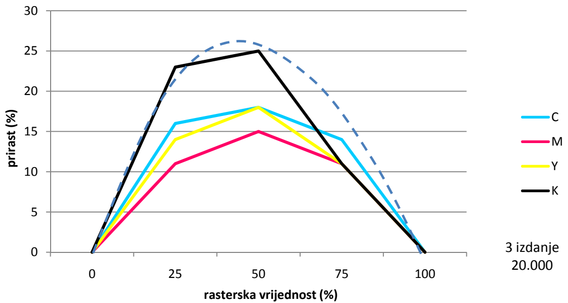
Graf 32. Prikaz krivulje prirasta rastertonskih vrijednosti na 25.000 -tom uzorku, 3 izdanja otisnutog na prvom tornju
