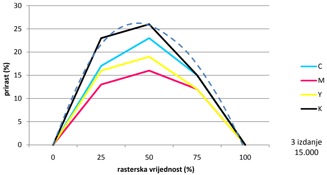
Graf 31. Prikaz krivulje prirasta rastertonskih vrijednosti na 15.000 -tom uzorku, 3 izdanja otisnutog na prvom tornju
