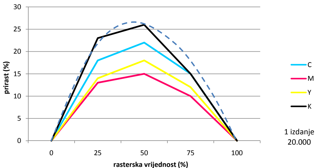
Graf 24. Prikaz krivulje prirasta rastertonskih vrijednosti na 20.000 -tom uzorku, 1i2 izdanja otisnutog na prvom tornju
