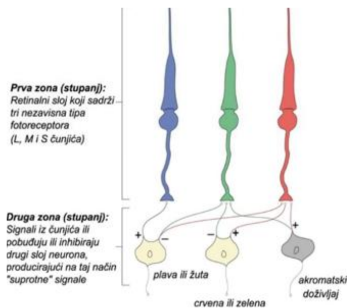
Slika 19. Prikaz prijenosa signala čunjićima u zonskoj teoriji viđenja boje [65]
