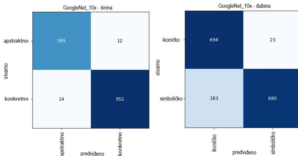
Slika 4. Matrice zbuđenosti (eng. confusion matrix) dviju fino ugođenih GoogleNet mreža, procijenjenih na potpuno novom validacijskom uzorku
