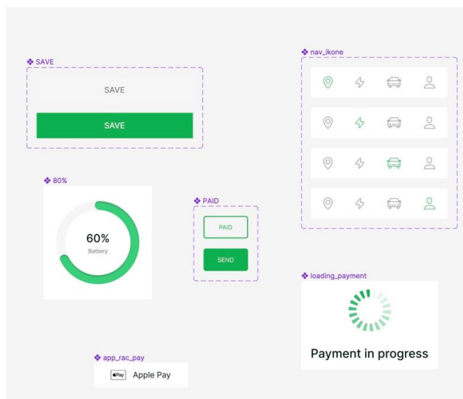
Slika 31: Atomi
