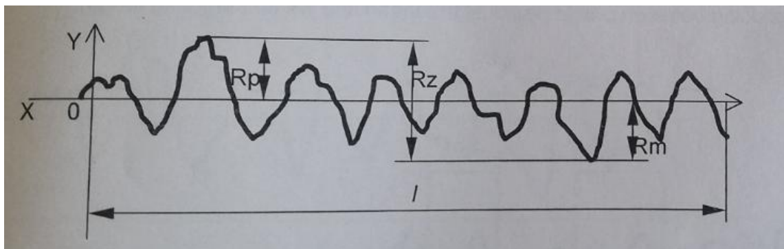
Slika 24. Maksimalna visina profila R_z
